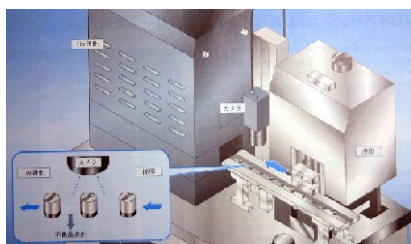
按印装置的文字质量检查
