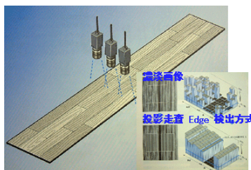
地板材料的宽度检查
