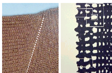
针孔位置的检出
