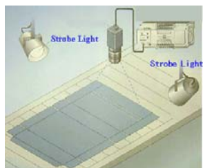
纸板上穿孔的有无检查
